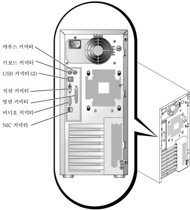
그림 B-1. I/O 포트 및 커넥터
