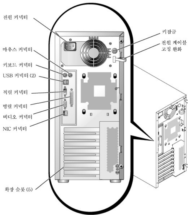
그림 1-3. 후면 패널 구조
